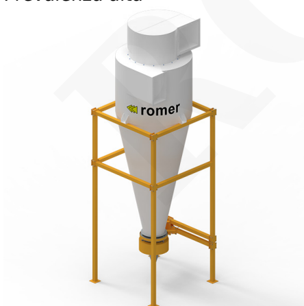
Separatori a ciclone
